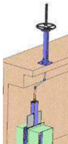
Карданное сочленение
