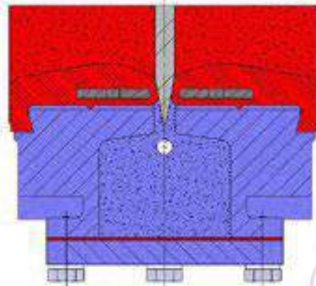
Секция D-D
