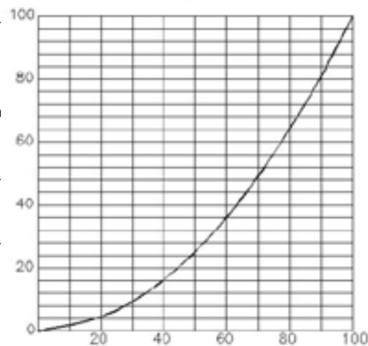
Вертикаль: % максимального расхода. Горизонтальный: %открытия клапана (квадратная диафрагма)
