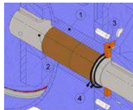
Кольцевые прокладки
