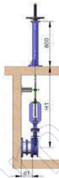
Стандартная колонна
