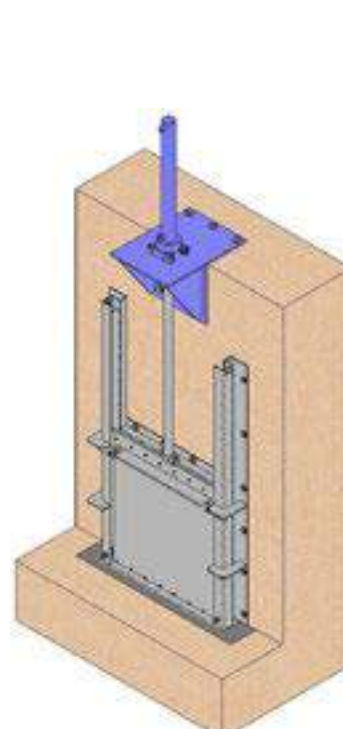
С гидроцилиндром
