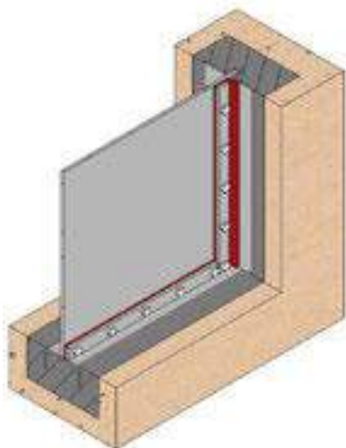
Бетонирование в дно и стенки
