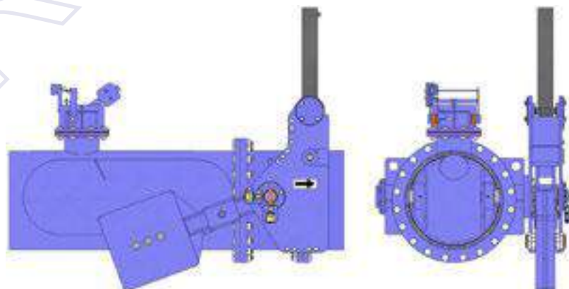
Датчик повышенной скорости активируется под действием потока → Дисковая задвижка закрывается.
