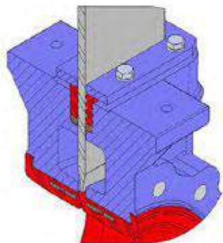
Деталь G
