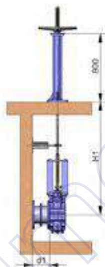
Стандартная колонна
