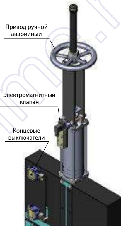
Ручной аварийный привод
