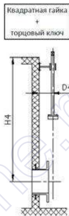
4. Аналогично 3+ торцовый ключ
