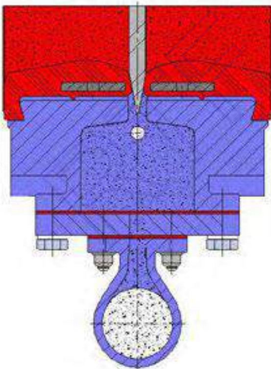
Секция E-E
