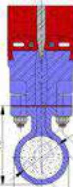
Секция B-B
