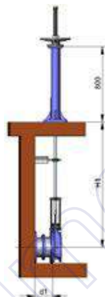
Стандартная колонна
