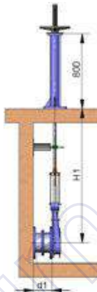
Стандартная колонна
