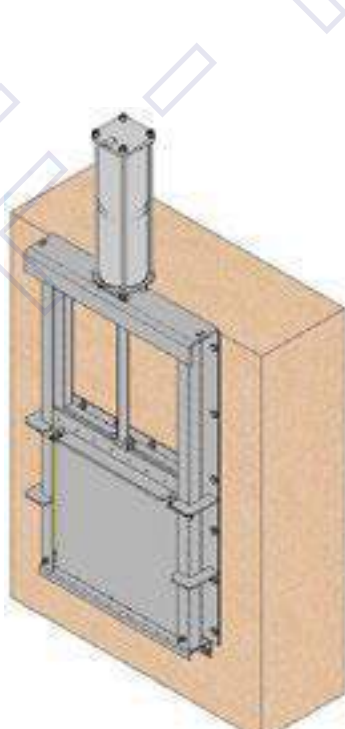
С пневмоцилиндром
