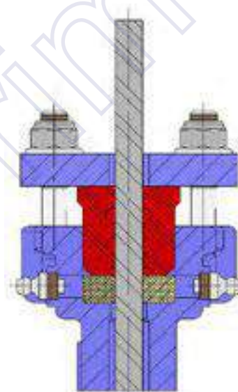
Секция F-F
